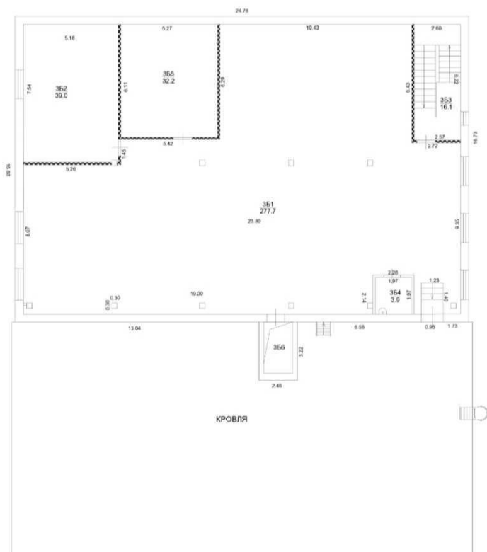
План этажа
