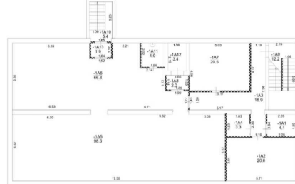
План этажа
