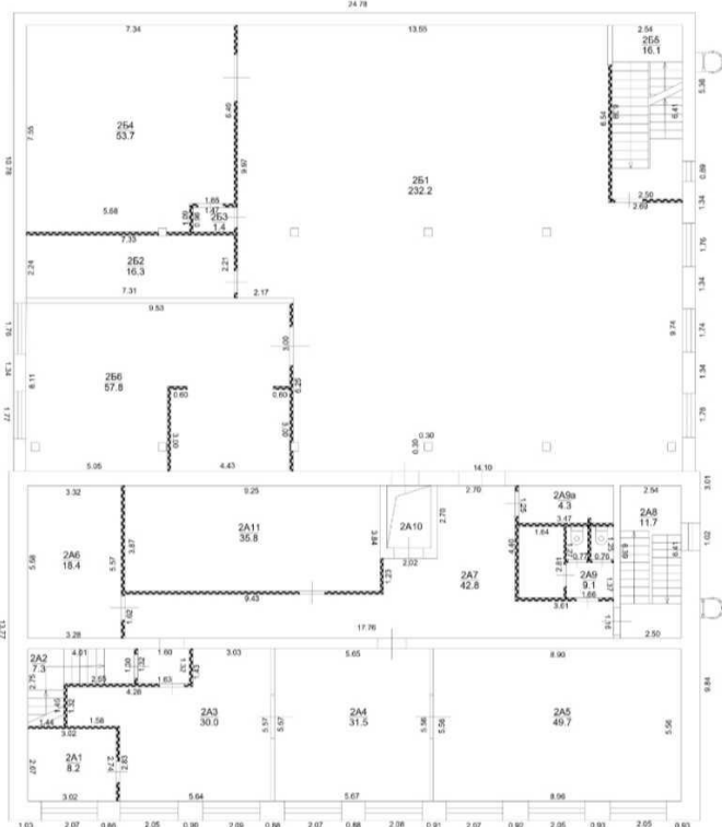
План этажа
