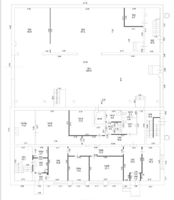
План этажа
